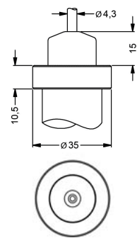
cable gland PG7 / cable length specify (IP 67) 2
